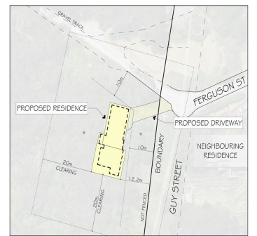
SITE PLAN 1:500
